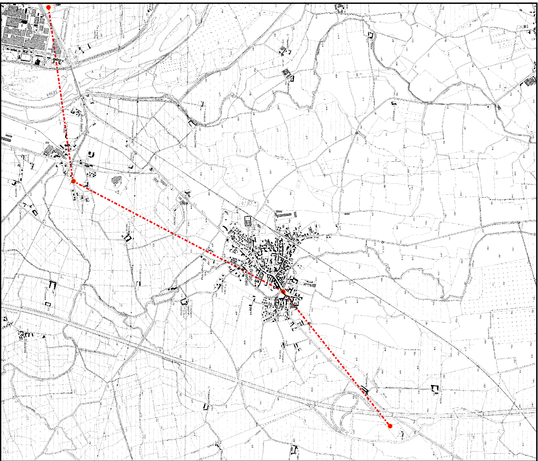
Scala 1:25.000 - Traccia della sezione litostatigrafica
